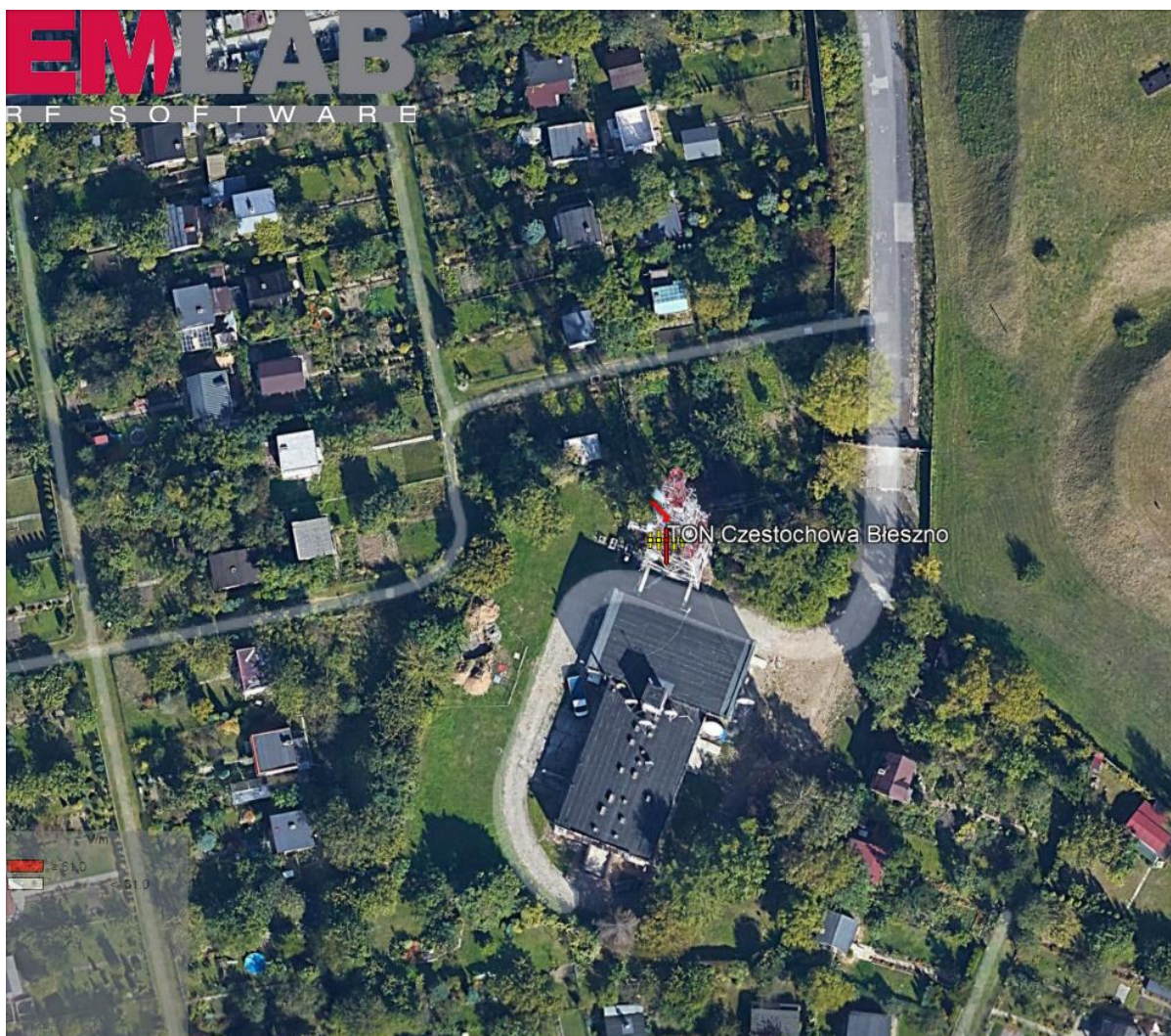
Rys. 2. Rzut poziomy rozkładu pola elektromagnetycznego anteny nowo projektowanej linii radiowej w otoczeniu TON Częstochowa / Bleszno przewidzianej do zainstalowania na wysokości 37 m nad poziomem terenu.
