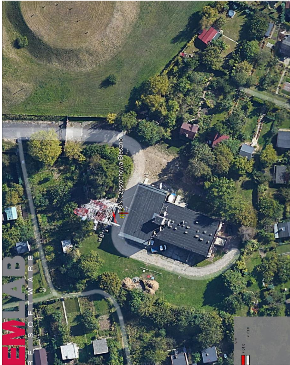
Rys. 2. Rzut poziomy rozkładu pola elektromagnetycznego anteny nowo projektowanej linii radiowej w otoczeniu TON Częstochowa / Bleszno przewidzianej do zainstalowania na wysokości 44 m nad poziomem terenu.
