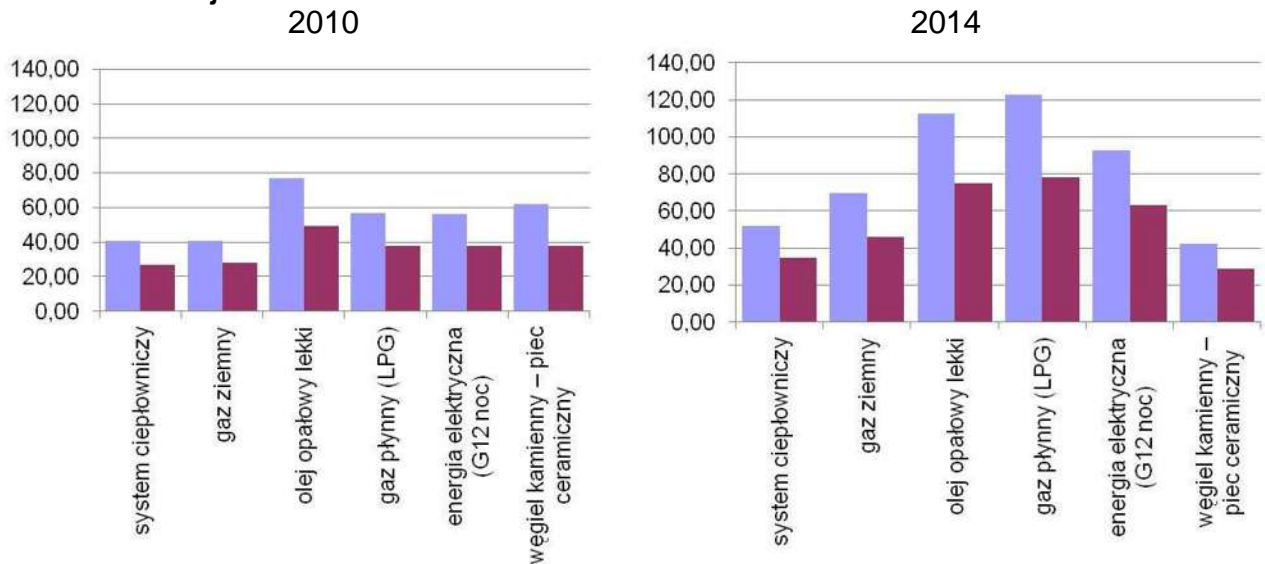
Wykres 11-1. Porównanie kosztów brutto nośnika energii [z /m 2 na rok] dla ogrzewania w zabudowie wielorodzinnej
