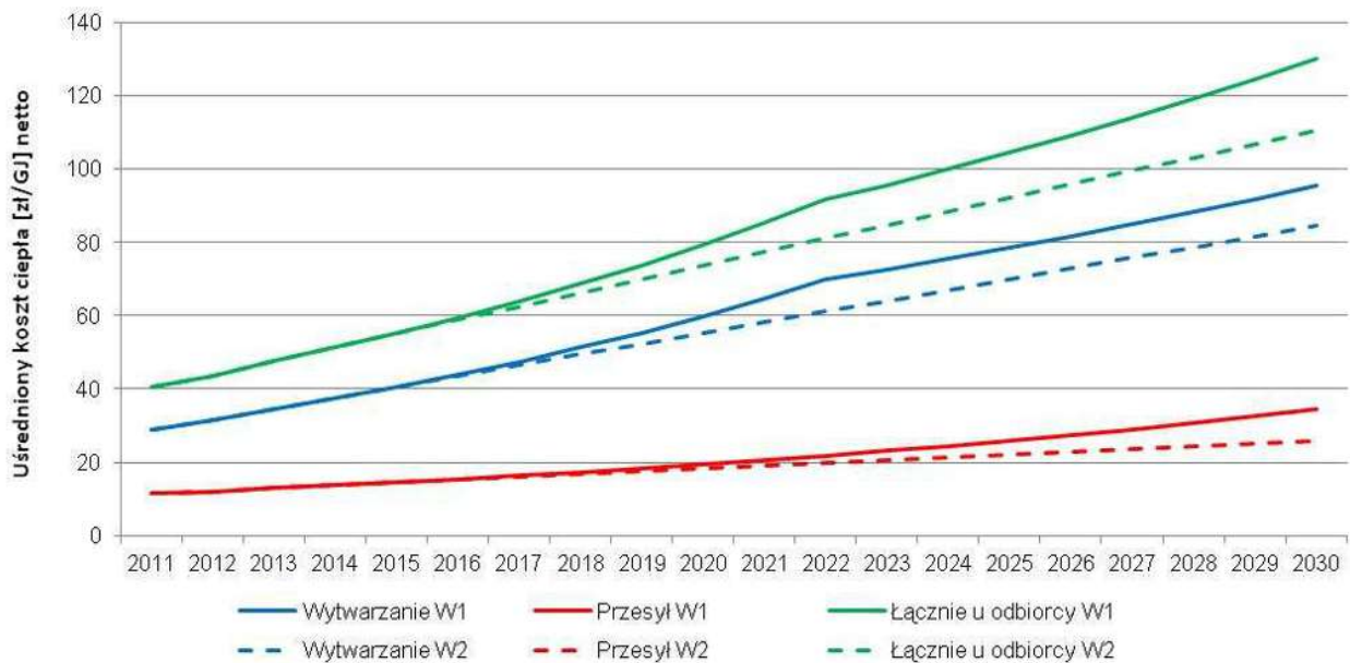
Wykres 10-4. Prognoza cen ciepła i systemowego w Częstochowie (ceny netto)
