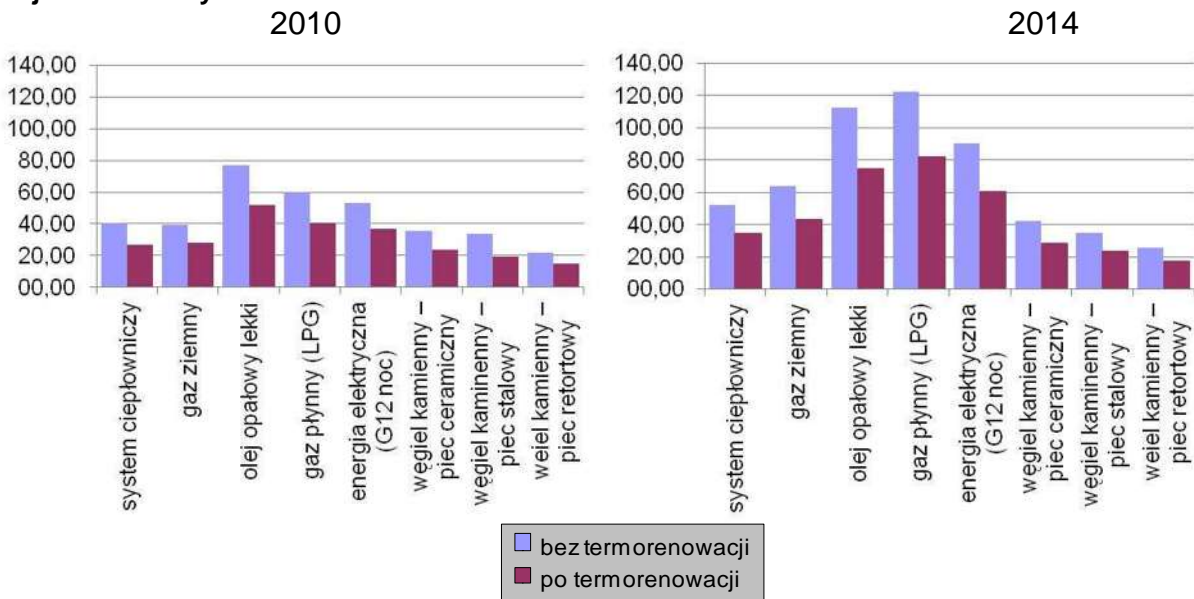
Wykres 11-2. Porównanie kosztów brutto nośnika energii [z /m 2 na rok] dla ogrzewania w budynku jednorodzinny
