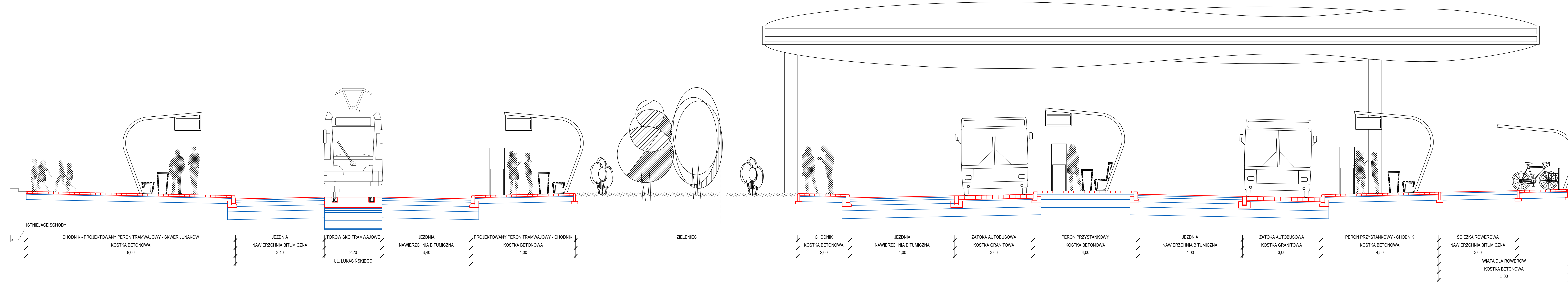
Przekrój typowy przez ul. Rejtana skala 1:50
