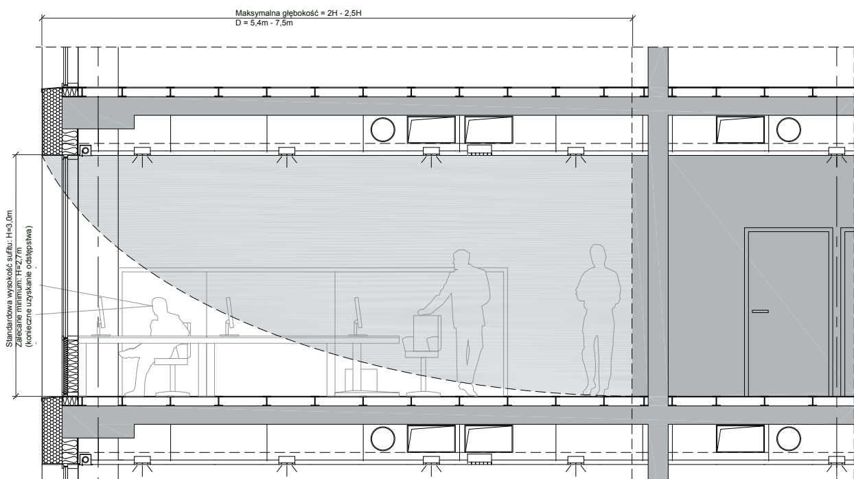
Zależność pomiędzy wysokością sufitu a głębokością pomieszczenia.
