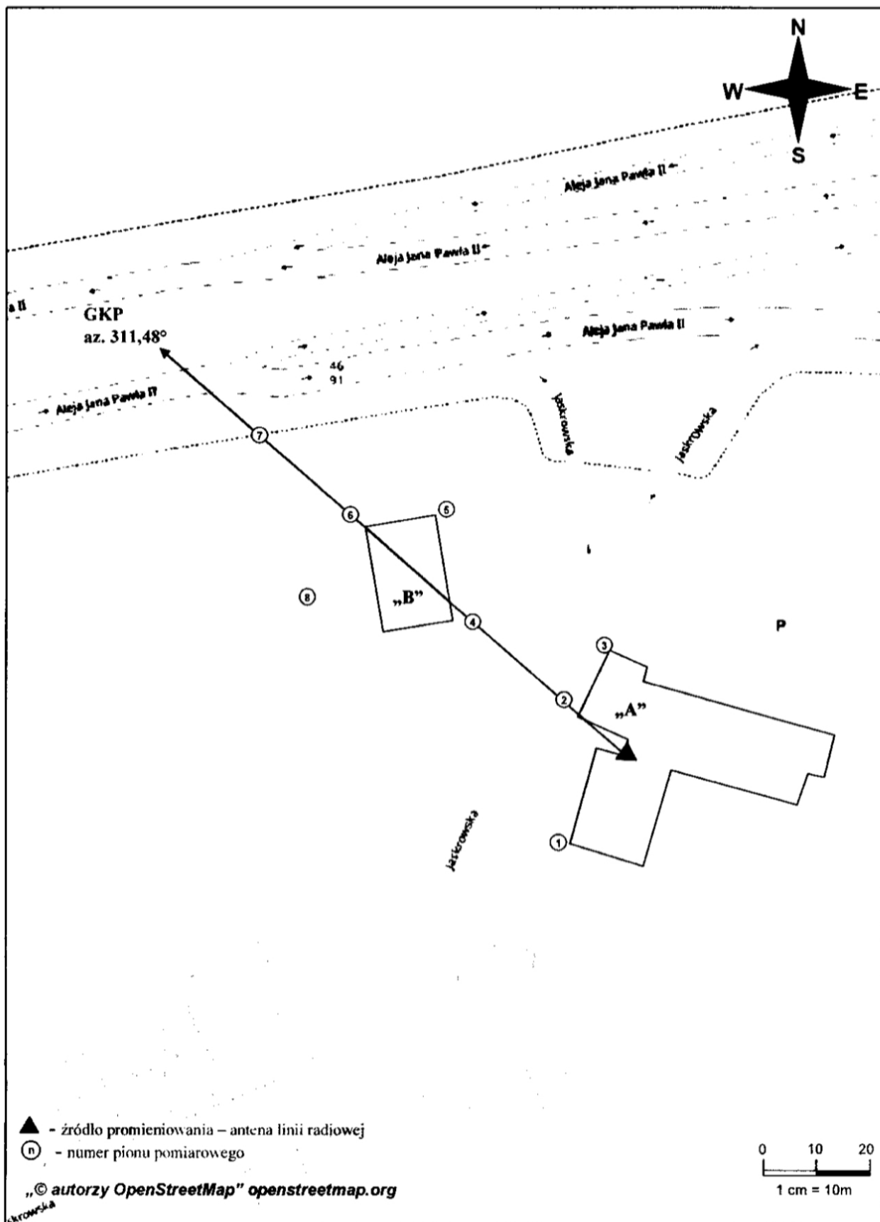
Rys. 1. Usytuowanie punktów i pionów pomiarowych w otoczeniu instalacji radiokomunikacyjnej Stacja Netia CZESB181-CZESM00081ANT002 Częstochowa, ul. Jaskrowska 22
